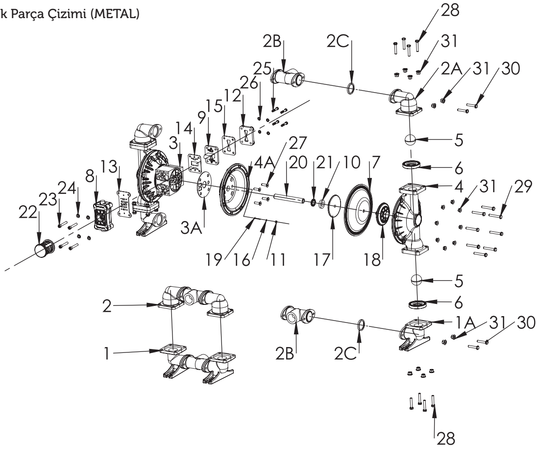
HP15 METAL GÖVDELİ POMPA PARÇA LİSTESİ
