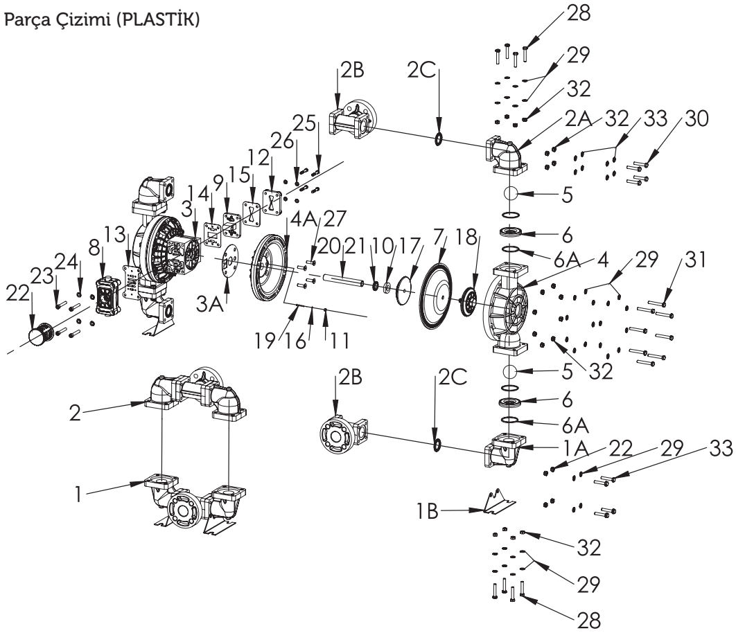
HP15 PLASTİK GÖVDELİ POMPA PARÇA LİSTESİ
