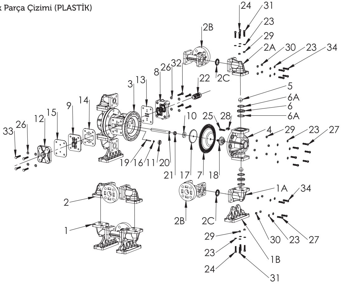
HP05 PLASTİK GÖVDELİ POMPA PARÇA LİSTESİ
