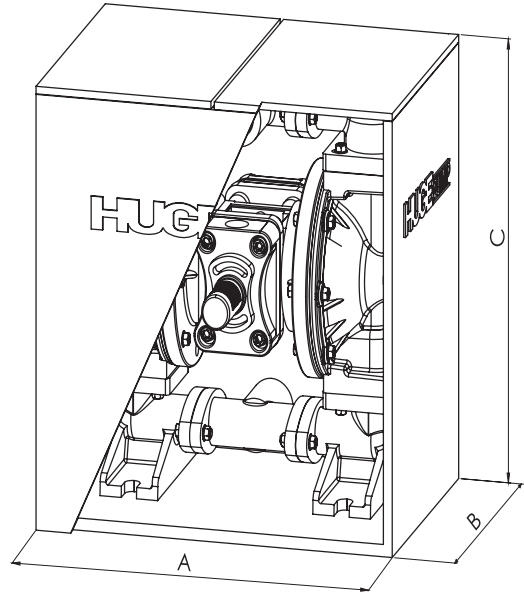
Metal Gövdeli Ölçülendirme
