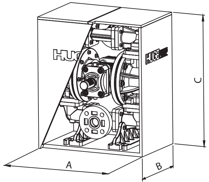
Plastik Gövdeli Ölçülendirme
