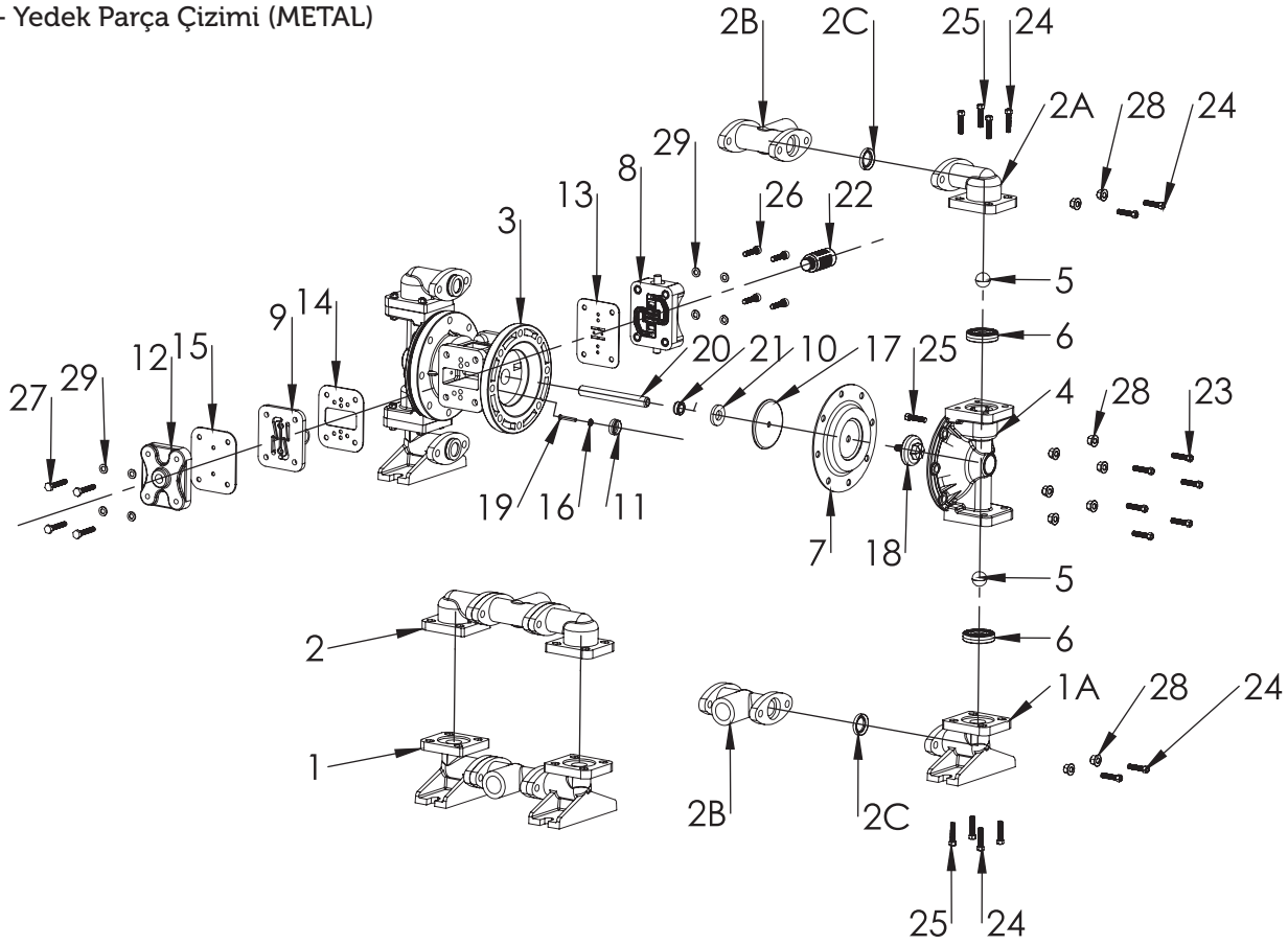
HP05 METAL GÖVDELİ POMPA PARÇA LİSTESİ
